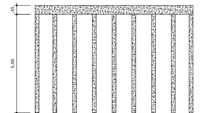
CORTE LONGITUDINAL
