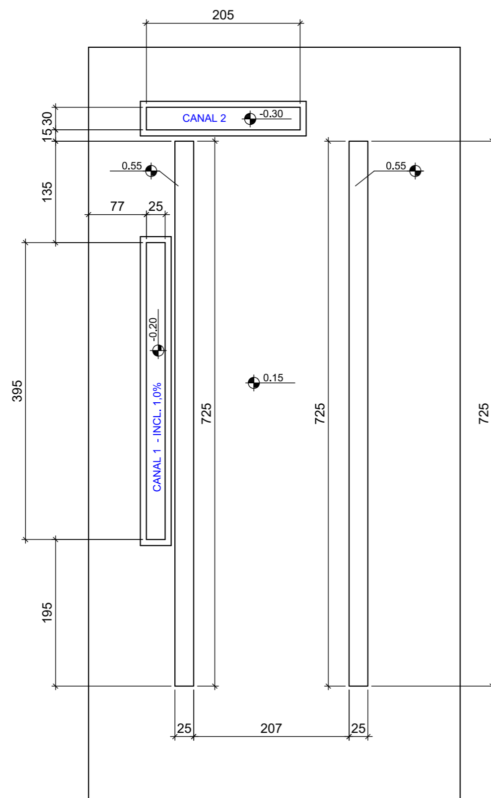
PLANTA DE BASES ESCALA 1:50
