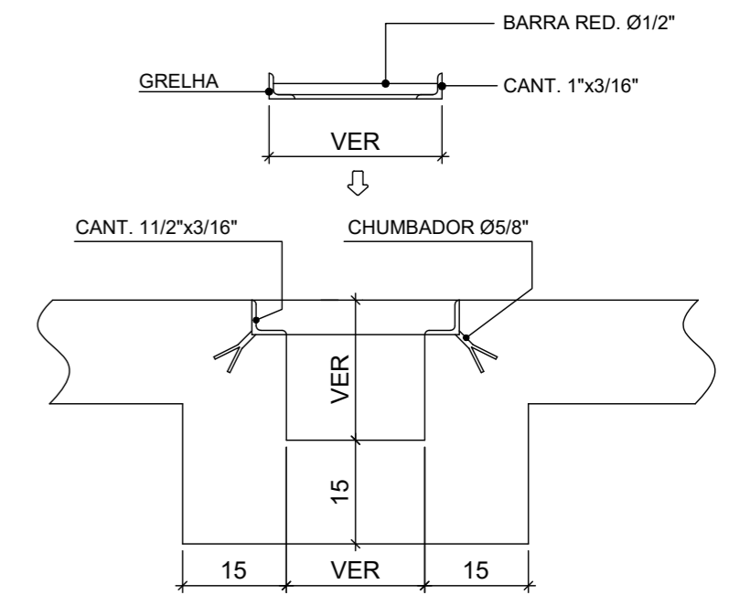
DETALHE TÍPICO DA CANALETA SEM ESCALA
