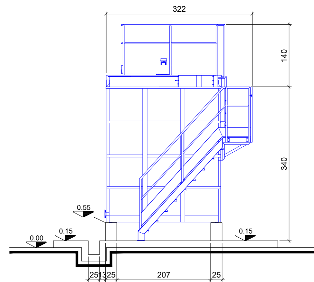
VISTA LATERAL ESCALA 1:50
