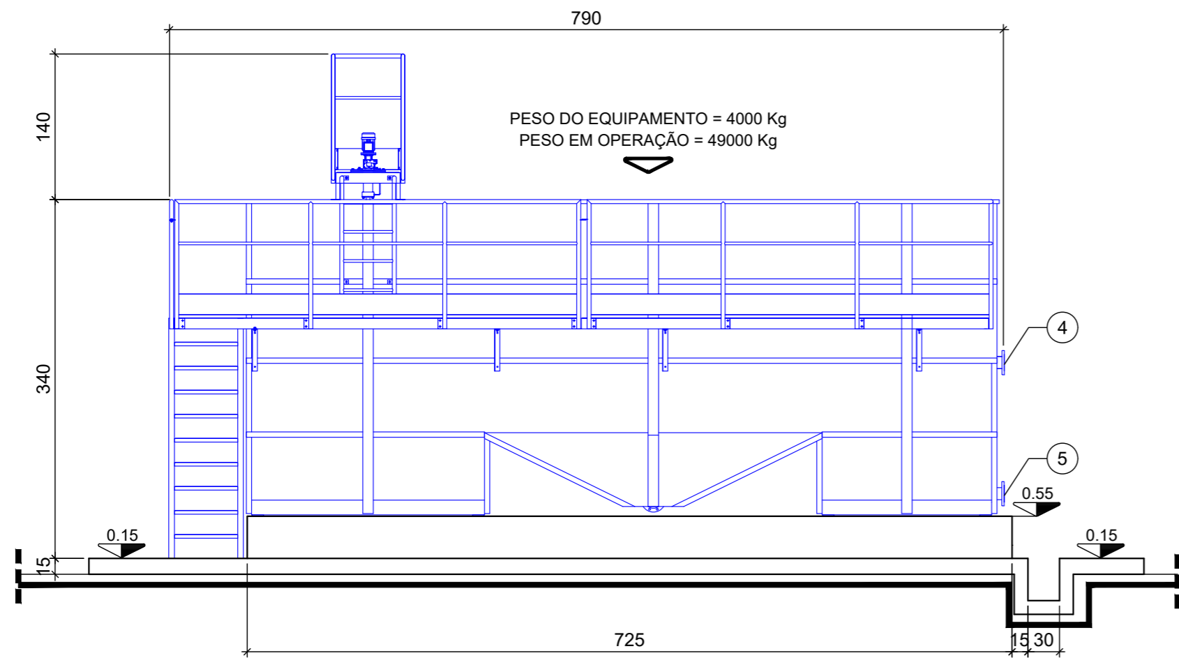
VISTA FRONTAL ESCALA 1:50
