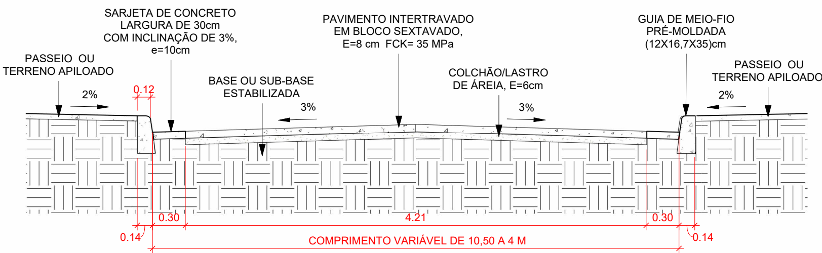
SEÇÃO TRANSVERSAL SEM ESCALA
