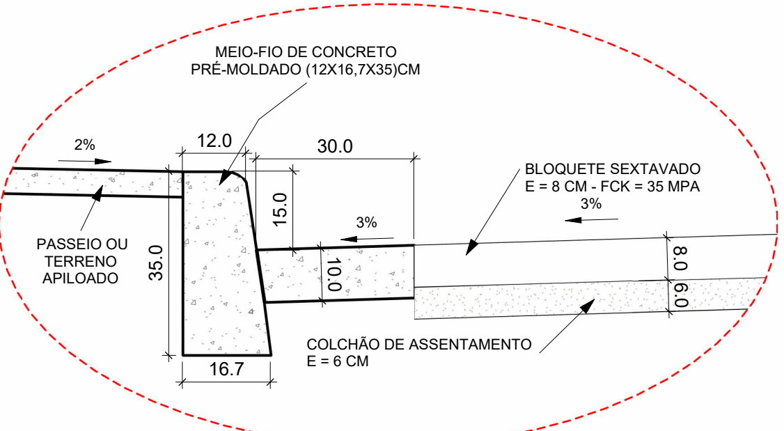
DETALHE SARJETA E MEIO-FIO SEM ESCALA
