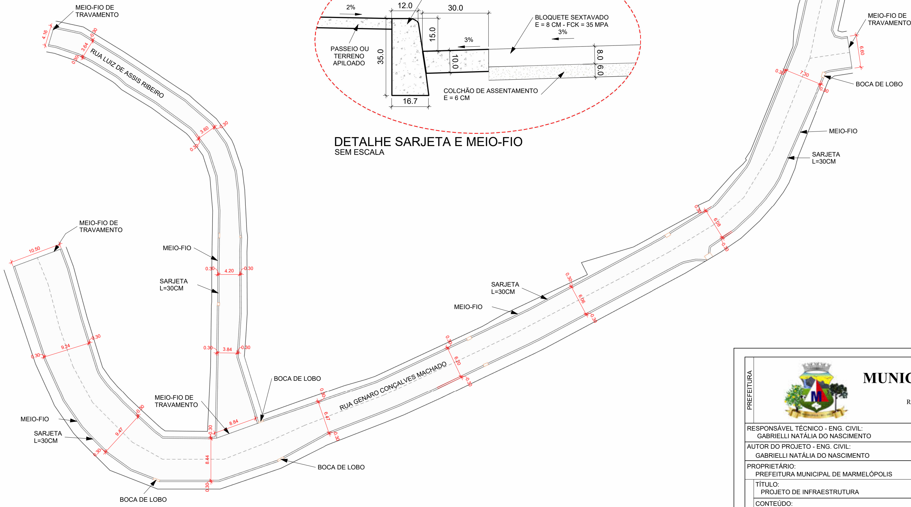
PLANTA DE CALÇAMENTO EM BLOQUETE SEXTAVADO ESC: 1 : 450
